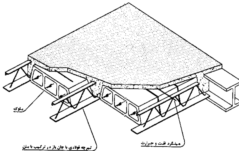
شکل (۱-۲) تیرچه فولادی، یا جان باز در ترکیب با بتن
