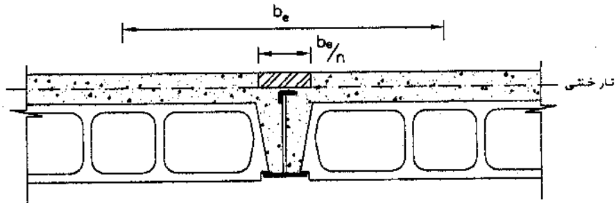
شکل (۳-۹) عرض موثر
